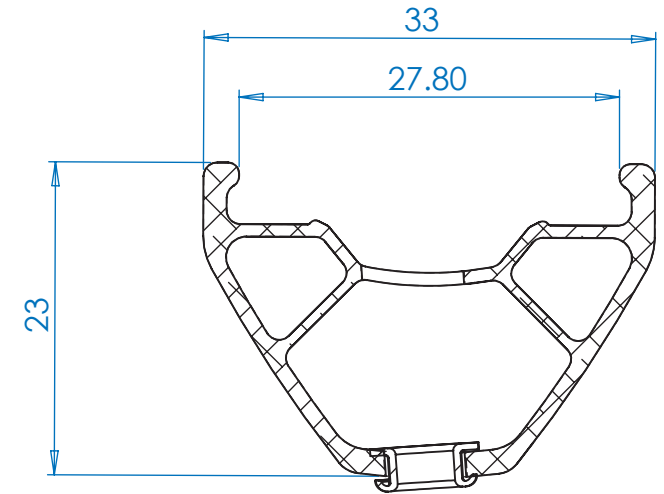
Tech DH Rim Profile
